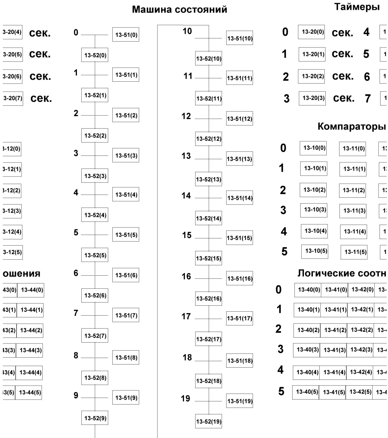
Рисунок 7.7 - Встроенный ПЛК ПЧВ3
